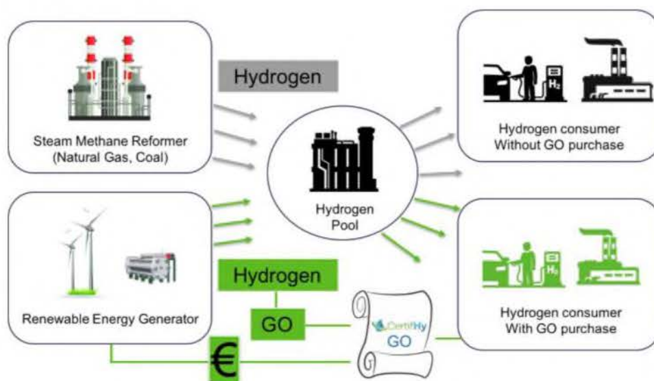
Obr. 4 - Koncepce záruky „zeleného“ původu vodíku 7
