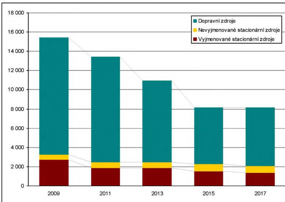
Trendy vývoje produkce emisí NO_x
