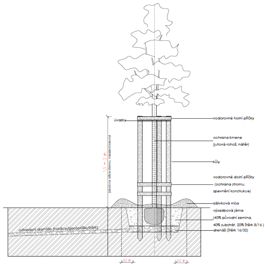
VZOROVÝ ŘEZ VÝSADBY STROMU, VČ. ODDRENÁŽOVÁNÍ
