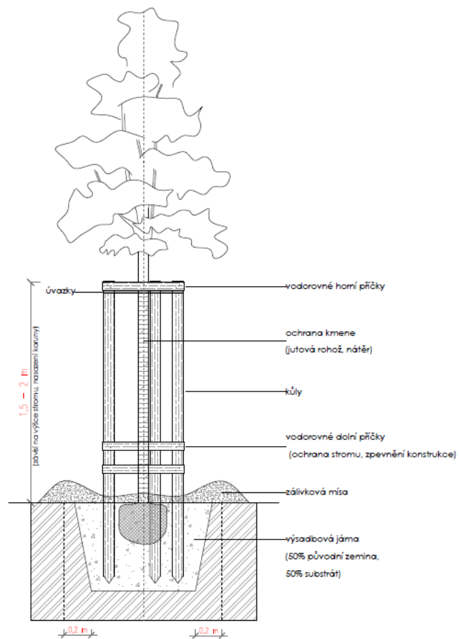
VZOROVÝ ŘEZ VÝSADBY STROMU
